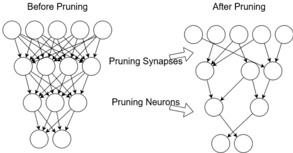
Figure : Illustration du Pruning dans un Réseau de Neurones
