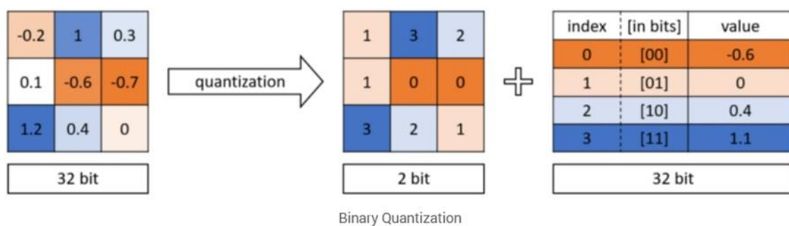
Figure : Illustration du processus de quantification binaire
